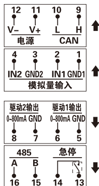
60系列—6080接收器接线端子功能定义:
